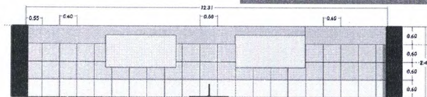
ELEVATION 1
