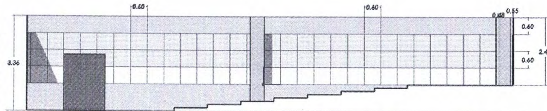
ELEVATION 1
